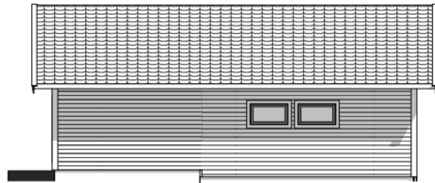
1:100 Fasade Øst
